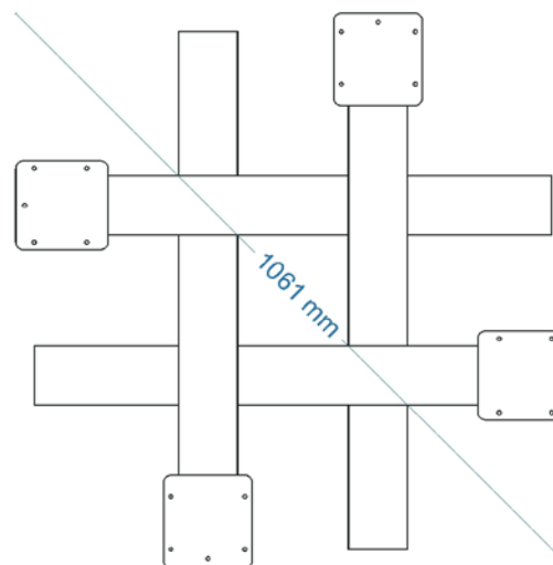
Widok z góry - długość przekątnej
