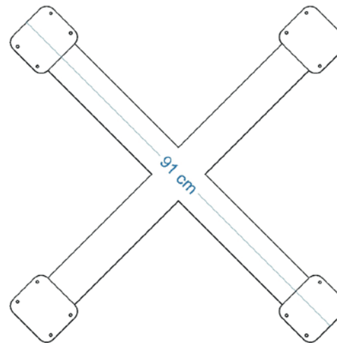
Widok z góry - długość przekątnej
